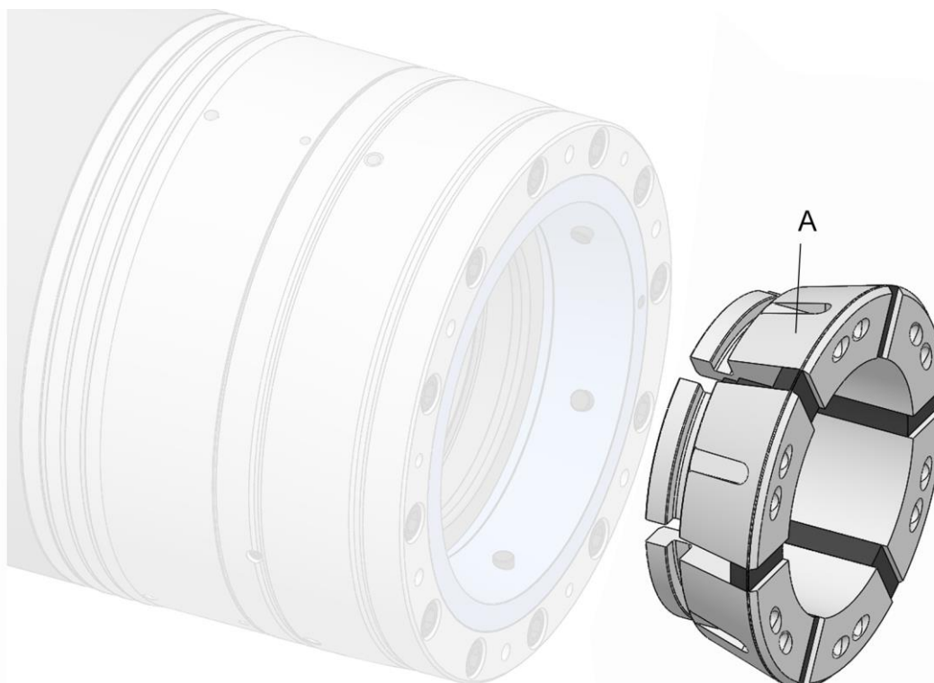
A Cabezal de sujeción [elemento de sujeción]
